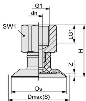
Конструктивные данные SGPN 30 NK-40 G1/4-IG
