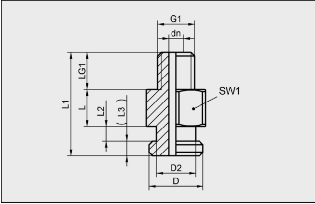
Tasarım verileri SA-NIP N028 M5-AG DN200
