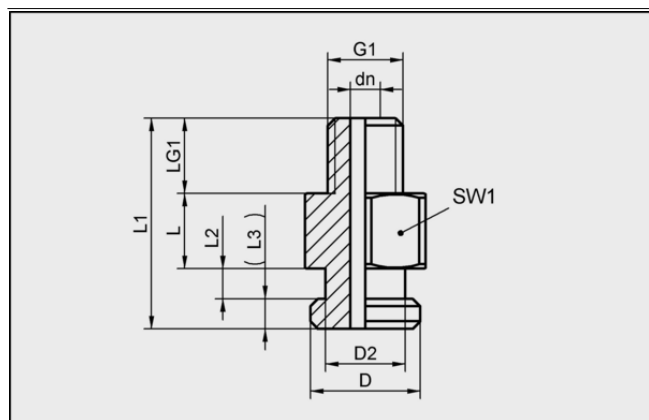
Données de construction SA-NIP N028 M5-AG DN200
