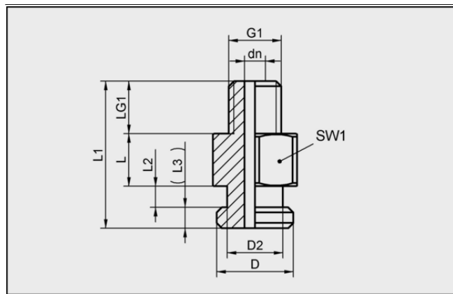
デザインデータ SA-NIP N028 M5-AG DN200
