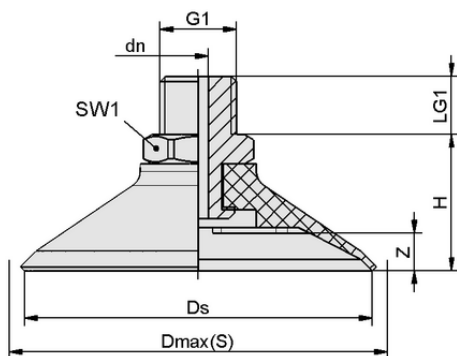
Конструктивные данные PFYN 60 VU1-72 G1/4-AG
