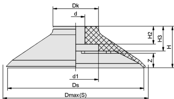
Dati di costruzione PFG 60 VU1-72 N011
