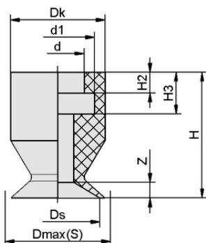
Dati di costruzione SGA 16 PU-55 N029
