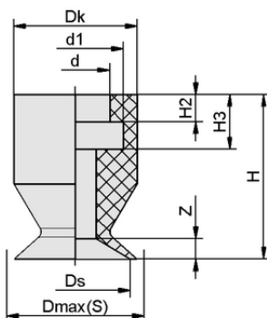
Données de construction SGA 9 PU-60 N028
