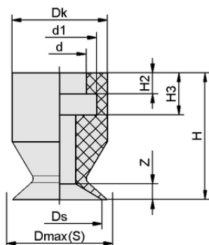
Конструктивные данные SGA 9 PU-60 N028
