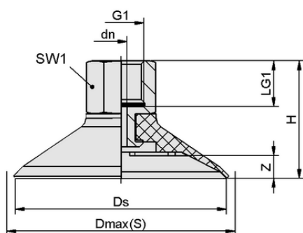
Конструктивные данные PFYN 15 VU1-72 G1/8-IG
