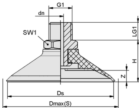
Datos de diseño PFYN 15 VU1-72 G1/8-AG
