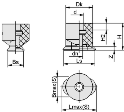
Datos de diseño SGO 7x3.5 NBR-55 N003
