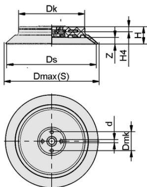
Конструктивные данные PFG 120 FPM-65 N010
