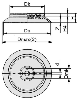
Datos de diseño PFG 120 FPM-65 N010
