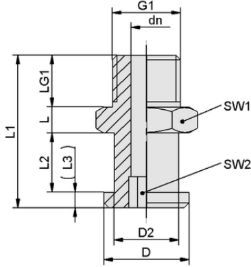
Tasarım verileri SA-NIP N003 M3-AG DN100
