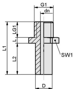
Конструктивные данные SA-NIP N001 M3-AG DN40
