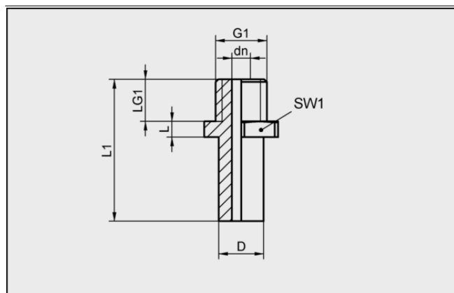
Конструктивные данные SA-NIP N002 M3-AG DN70
