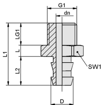
Конструктивные данные SA-NIP N020 M5-AG DN180
