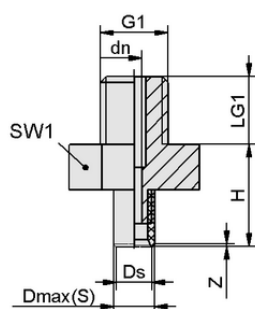
Конструктивные данные PFYN 1 SI-55 M3-AG
