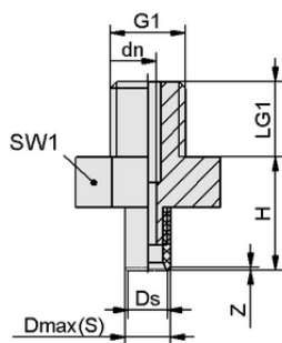
Конструктивные данные PFYN 1 NBR-55 M3-AG
