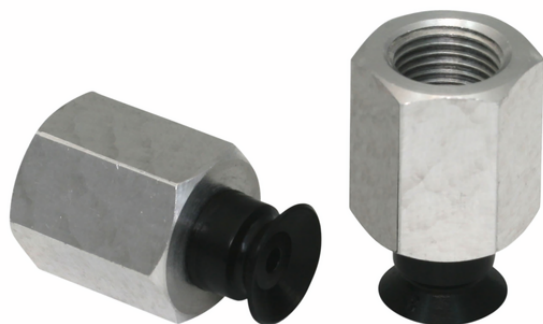
PFYN 10 NBR-55 G1/8-IG
