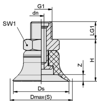
Конструктивные данные PFYN 15 NBR-55 G1/8-AG
