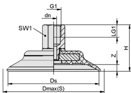
Конструктивные данные PFYN 95 FPM-65 G1/4-IG
