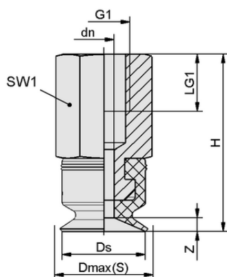
Конструктивные данные PFYN 10 SI-55 M5-IG
