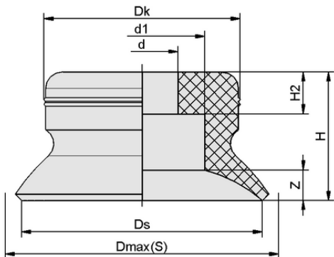
Datos de diseño PFG 40 FPM-65 N007
