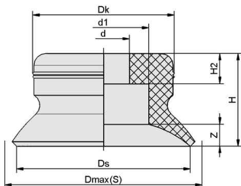
Dati di costruzione PFG 40 FPM-65 N007
