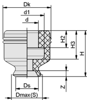
Datos de diseño PFG 6 FPM-65 N004
