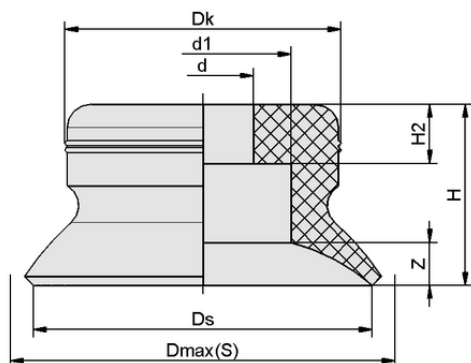
Конструктивные данные PFG 40 SI-55 N007
