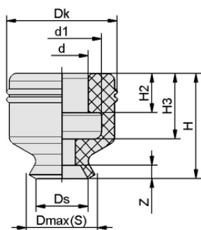
Конструктивные данные PFG 10 SI-55 N004
