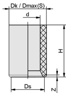
Конструктивные данные PFG 1 SI-55 N001
