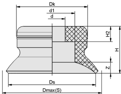
Données de construction PFG 40 NBR-55 N007
